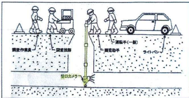
図 3-5 管口カメラ点検工の作業模式図
